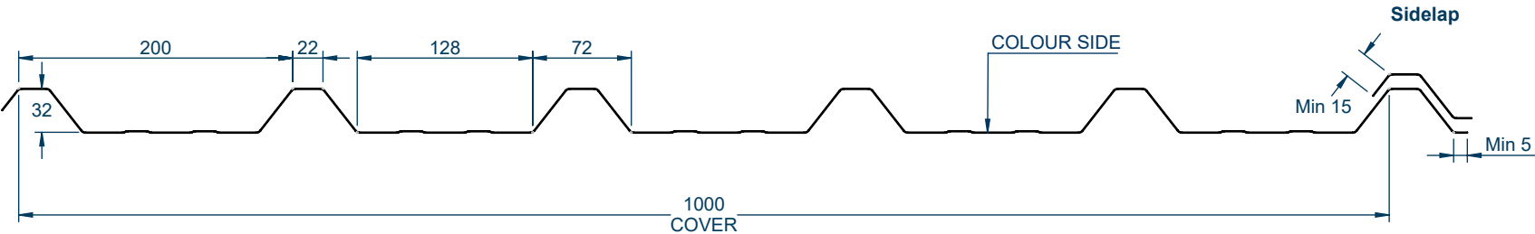
Sidelap
